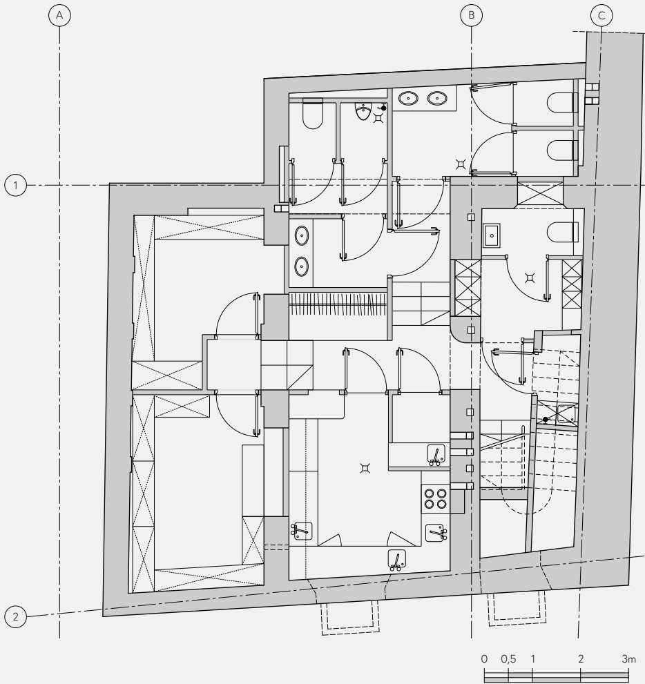
Rzut piwnicy
